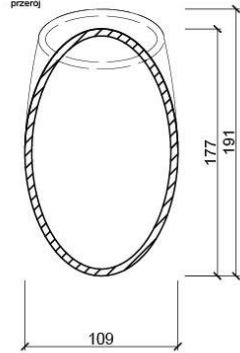
przerój
