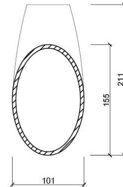
przerój
